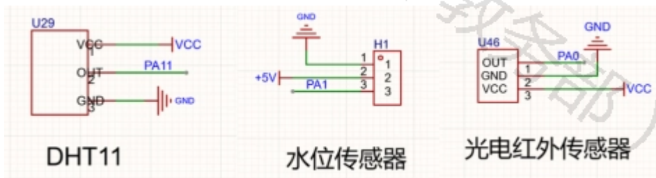
图17 状态采集模块电路原理图
