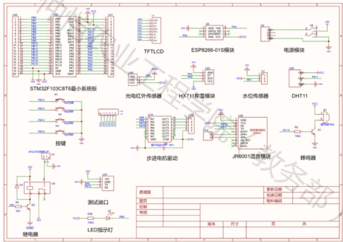
图15 原理图
