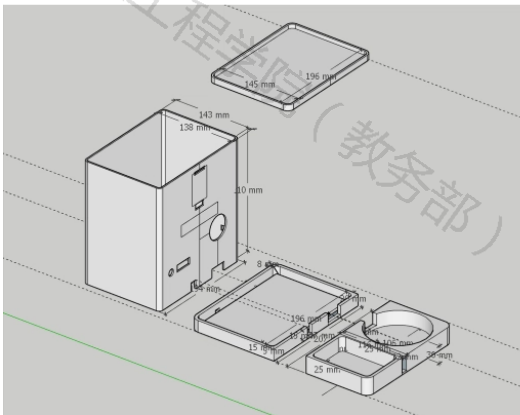
图13 SketchUp三维建模设计图视角a
