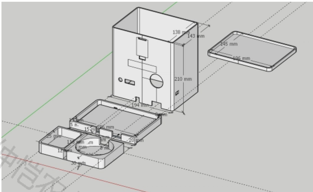
图13 SketchUp三维建模设计图视角a
