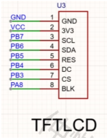
图20 通信与显示模块电路原理图
